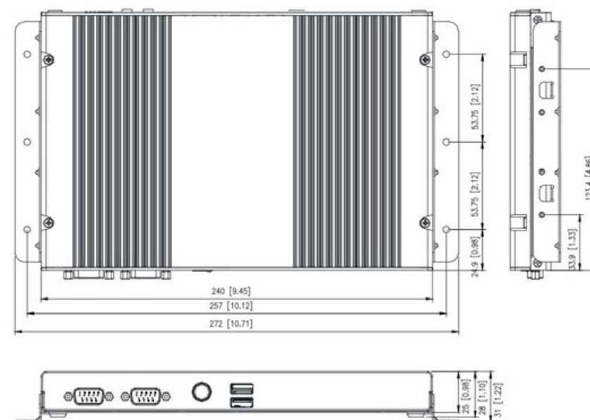
Dimensiones en mm y [pulgadas]
